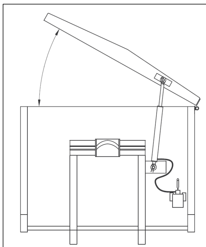
Figura 2 - ESEMPIO CASSONE CON APERTURA COPERCHIO CON CERNIERE A DESTRA
