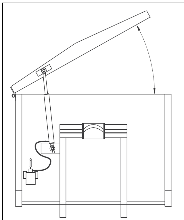
Figura 1 – ESEMPIO CASSONE CON APERTURA COPERCHIO CON CERNIERE A SINISTRA
